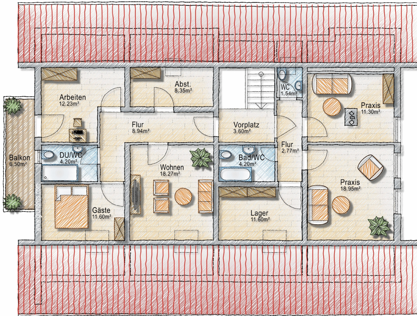
Dachgeschoss
